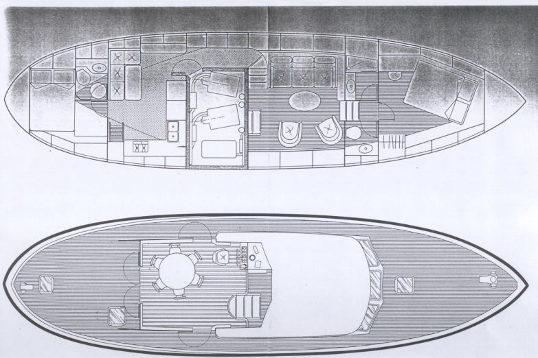
Motor Yacht 16,00 m 11 Postes - Fin 2003
